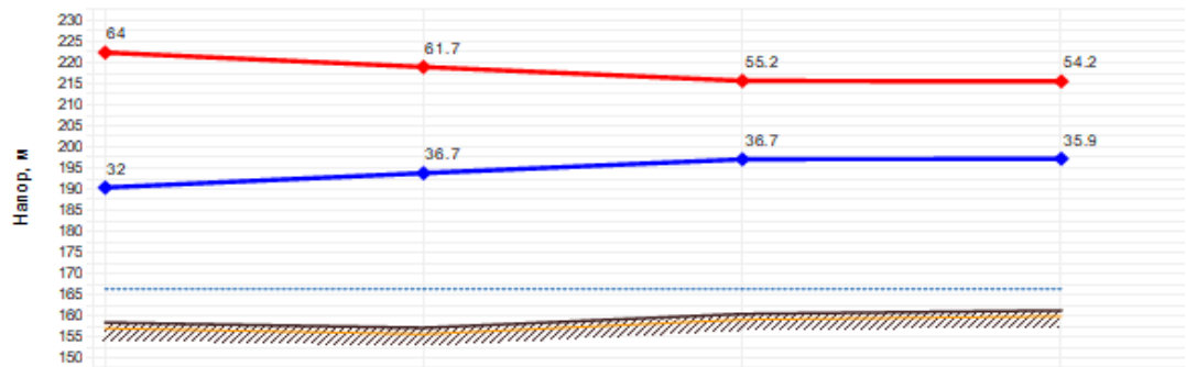
Пьезометрический график от «с. Отрадное, Октябрьская 33г» до «Школа»
