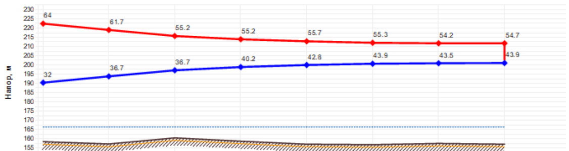
Пьезометрический график от «с. Отрадное, Октябрьская 33а» до «ул. Ленина д.4»
